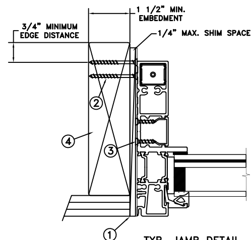
TYP. JAMB DETAIL HORIZONTAL SECTION
